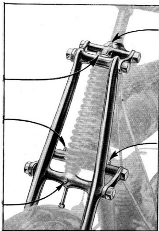
Fig. 19. — Graissage de la fourche de la 100 cm 3 .
