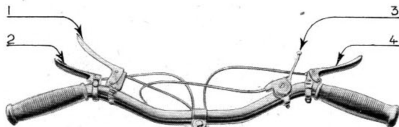
Fig. 11. — Guidon de la 100 cm 3
