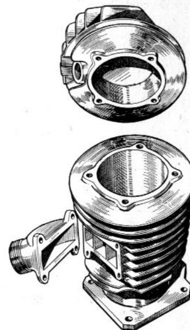
Fig. 14. — Moteur 175 cm 3 , cylindre avec culasse et pipe d'admission démontées pour le décalaminage.
