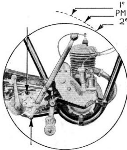
Fig. 15. — Graissage de la boîte de vitesses de la 175 cm 3 . Les flèches de gauche indiquent les bouchons de remplissage et de vidange. — En haut à droite, schéma de position des vitesses.
