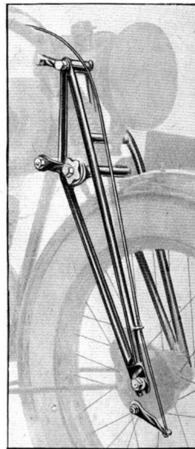
Fig. 18. — Vue de la fourche et de la commande du frein sur roue avant de la 308 cm 3 .
