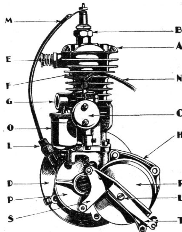
Fig. 1. — Moteur 100 cm 3 à volant magnétique.
