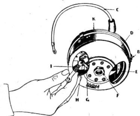
Fig. 16. — Volant magnétique NOVI (capot enlevé) Manière de régler l'écartement des vis platinées
