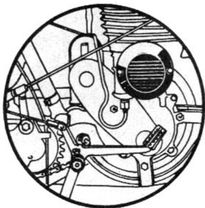
Fig. 19. — Filtre du carburateur de la 308 cm 3
