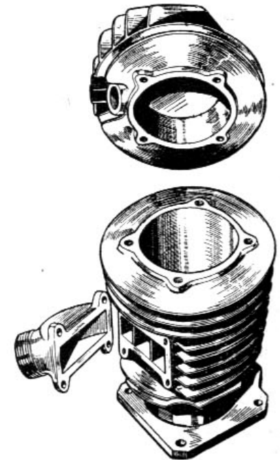
Fig. 11. — Moteur 175 cm 3 , cylindre avec culasse et pipe d'admission démontées pour le décalaminage.
