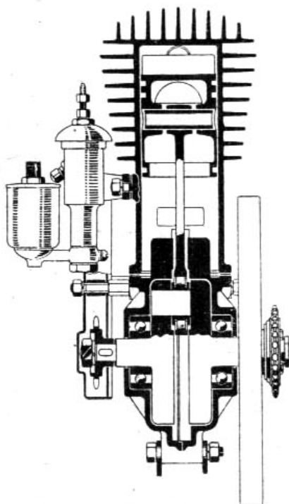
Fig. 5. — Coupe longitudinale du moteur 2 temps
