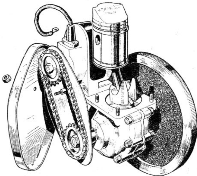
Fig. 10. — Moteur (type 175 cm 3 ), cylindre et culasse enlevés
