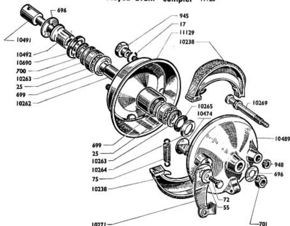
Moyeu avant complet 11128
