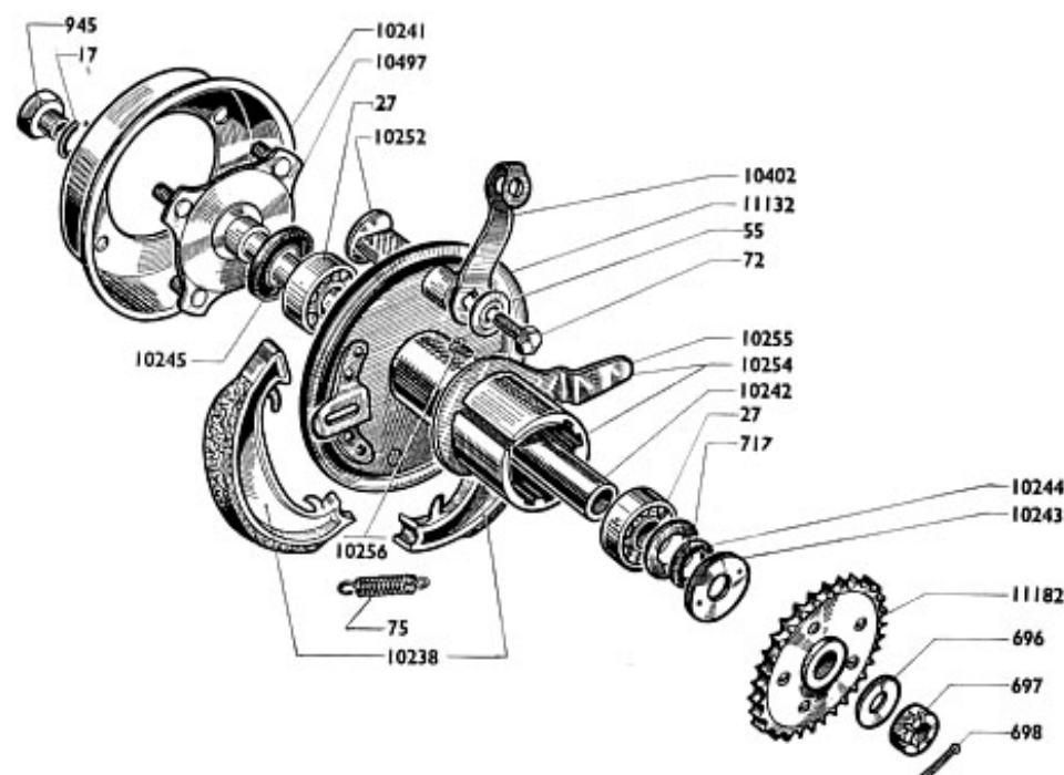
Moyeu arrière complet 11131
