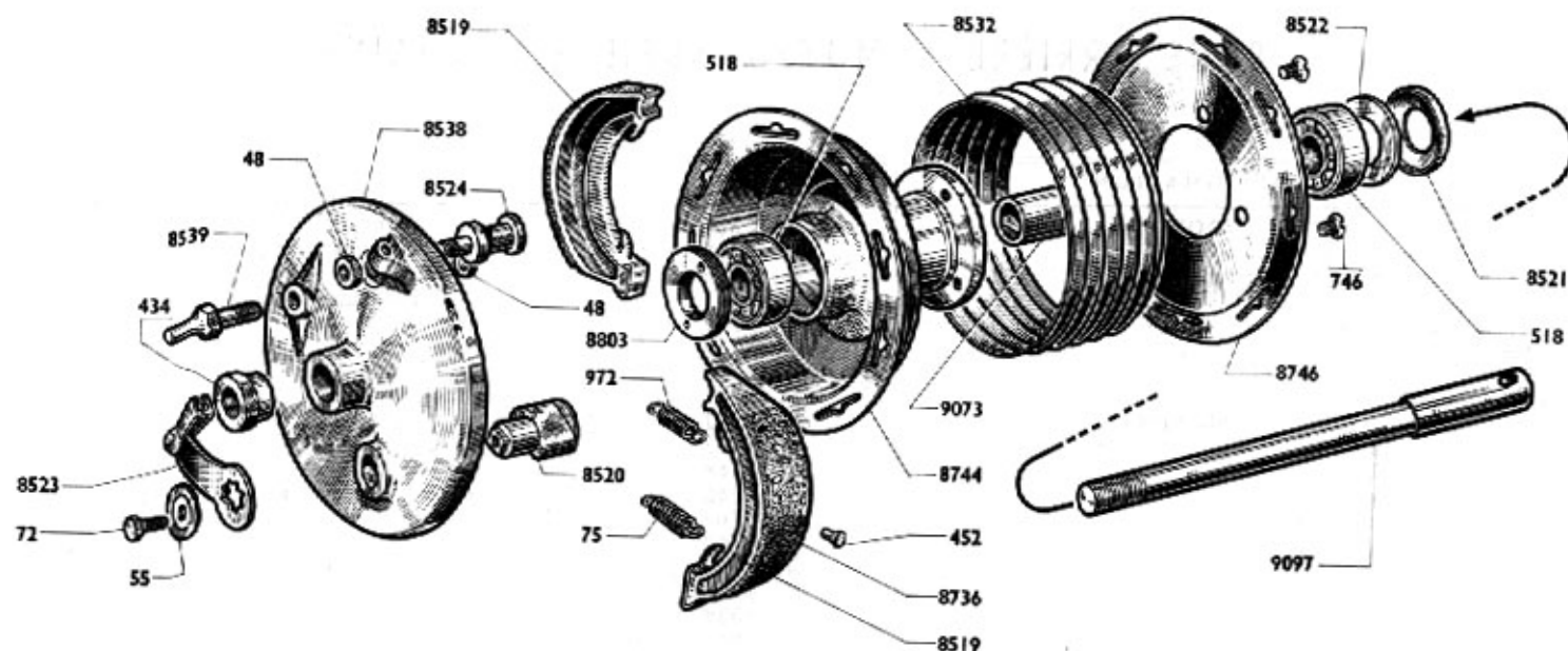
ROUE ET MOYEU AVANT
