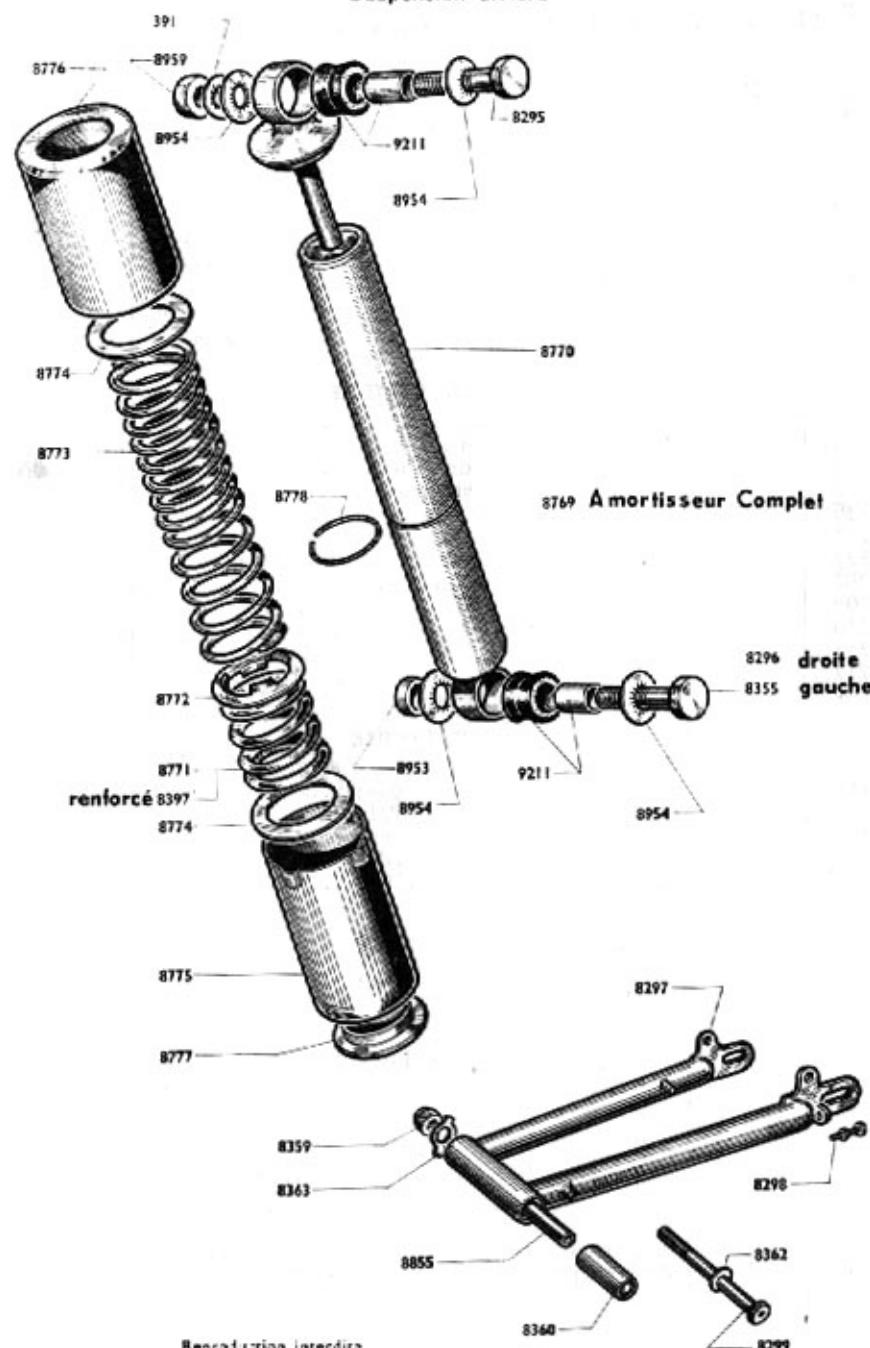
Suspension arrière
