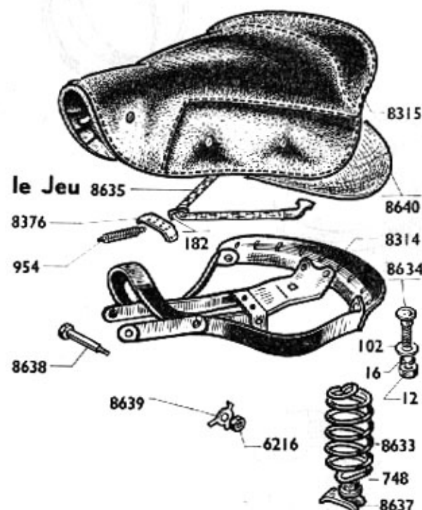
Selle complète mono-ressort 8313
