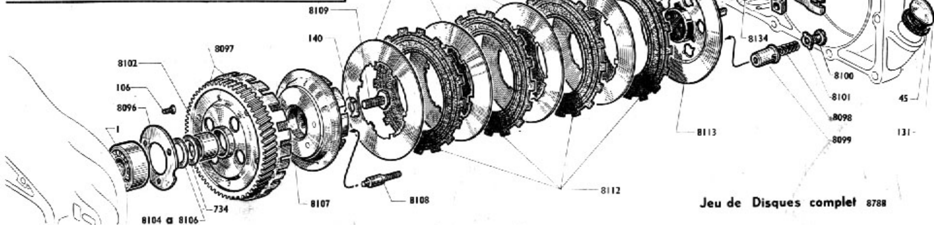
Embrayage Complet 8398
