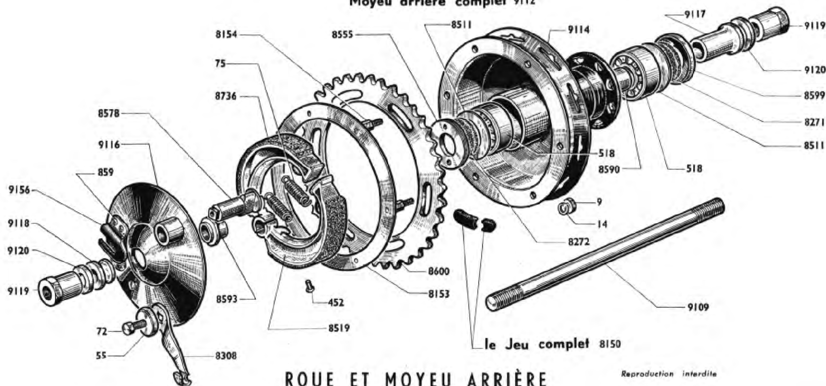
Moyeu arrière complet 9112
