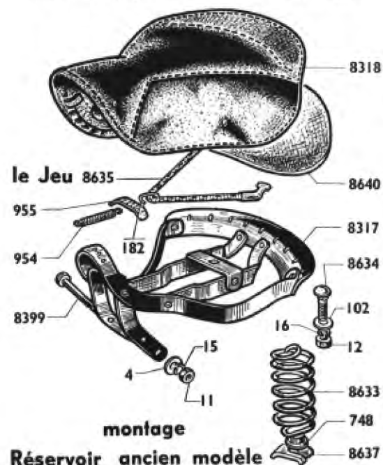
Selle complète mono-ressort 8316
