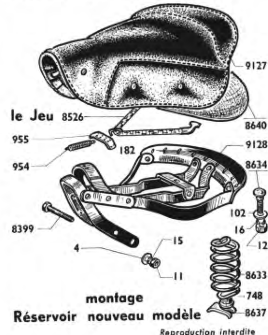
Selle complète mono-ressort 9126
