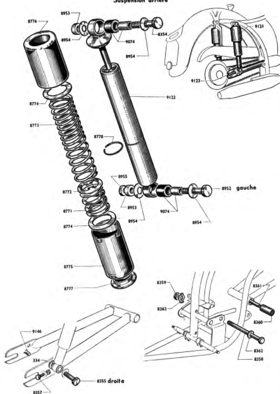
Suspension arrière
