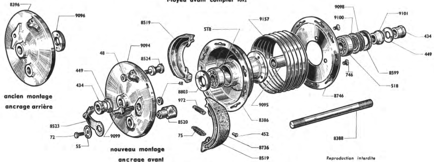
Moyeu avant complet 9092
