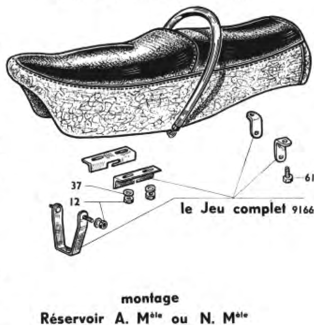
Selle Bi-place complète 9169
