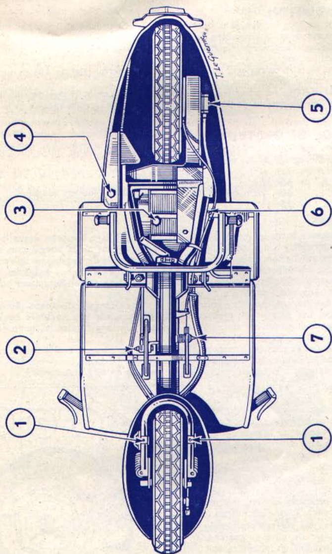
1. Graisseur du pont de fourche — 2. Graissage de pédale de sélecteur — 3. Bouchon de vidange de carter — 4. Bouchon de vidange de boîte à huile — 5. Graisseur prise de compteur — 6. Graisseur de câble de frein à main — 7. Graisseur de pédale de frein.
