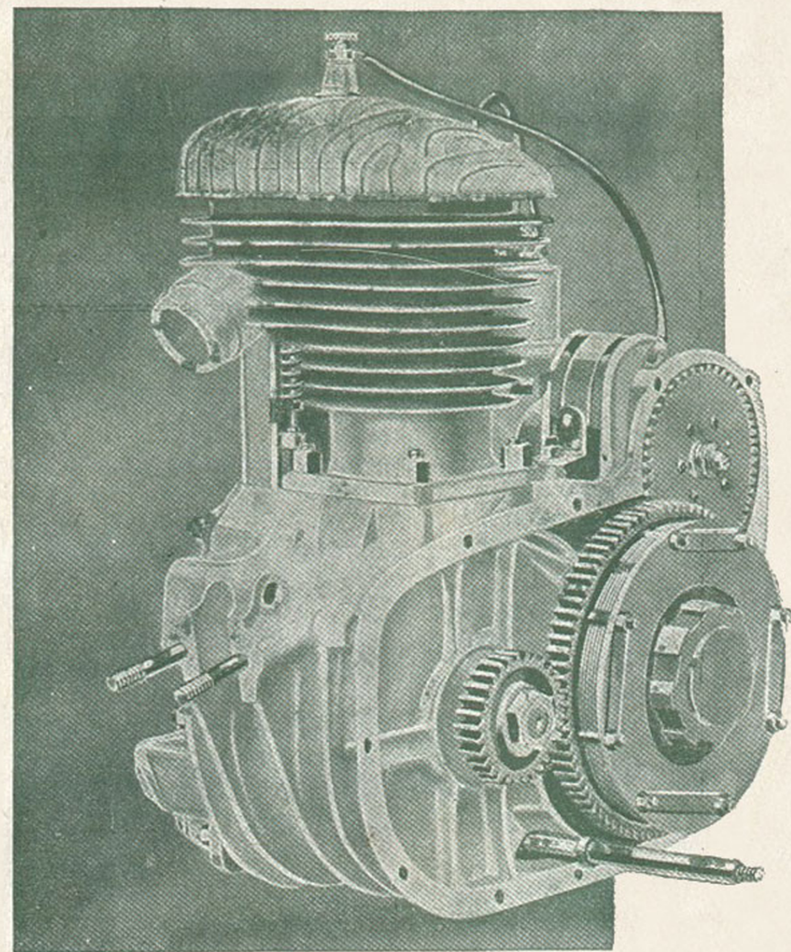
BLOC-MOTEUR Motoconfort
