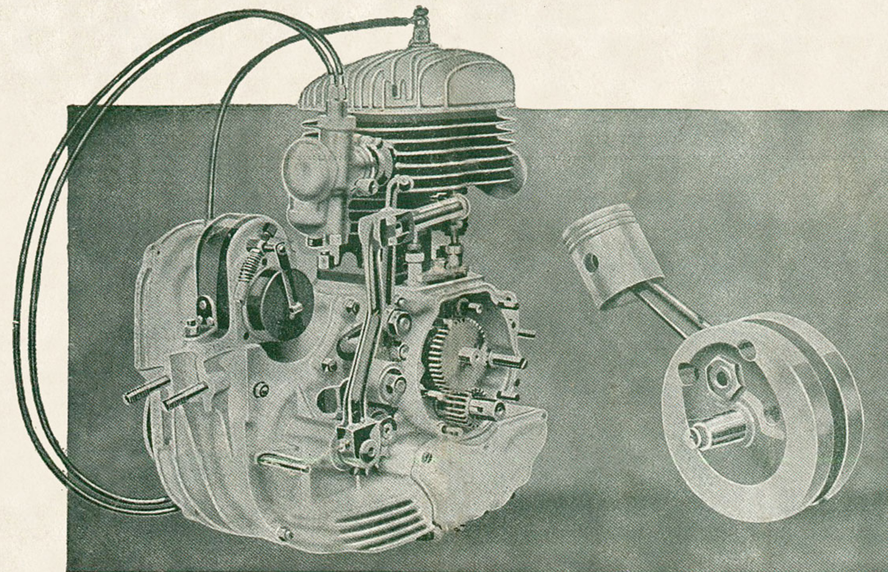
BLOC-MOTEUR Motoconfort 4 CV. 4 Temps
