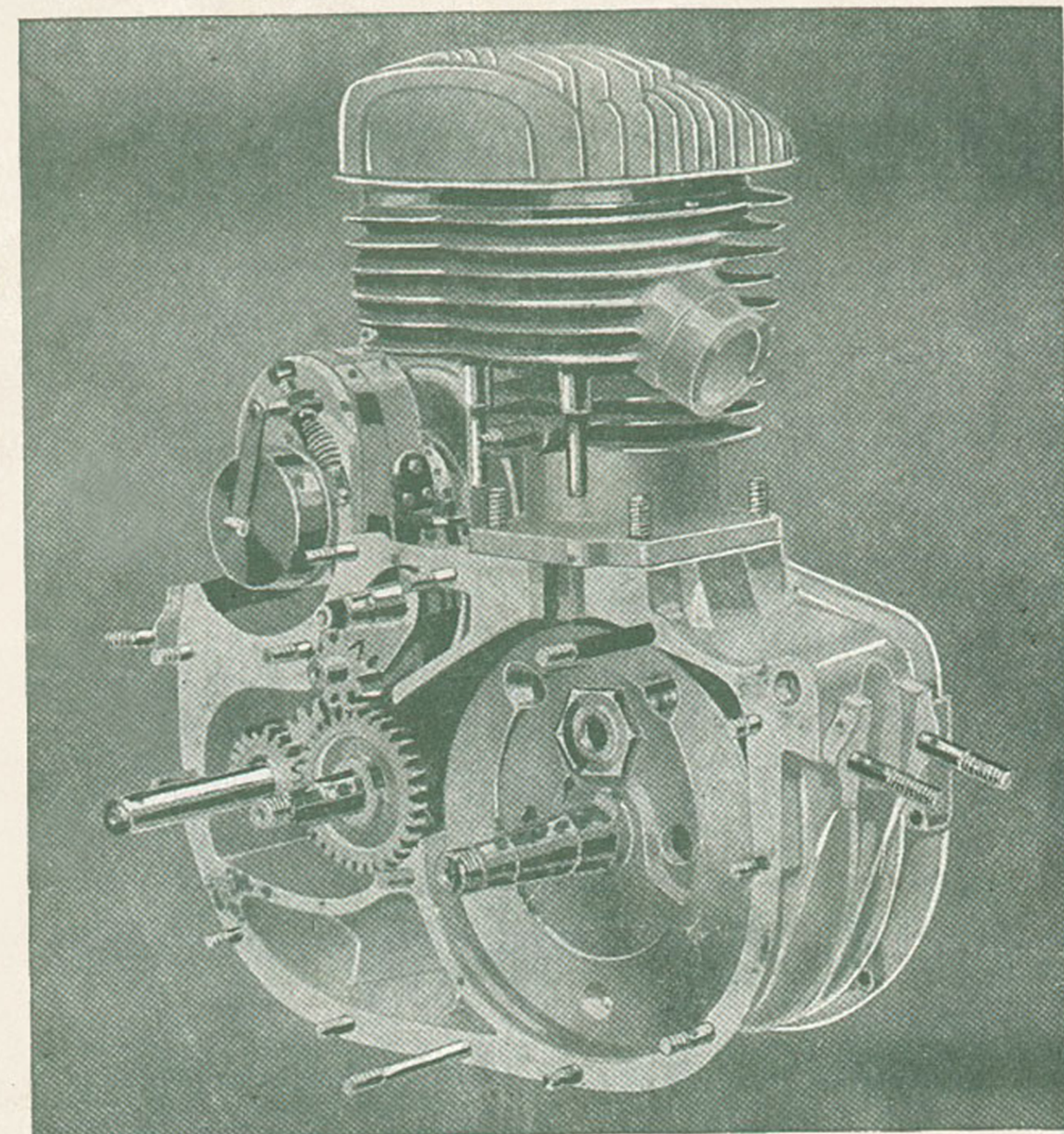
BLOC-MOTEUR Motoconfort
