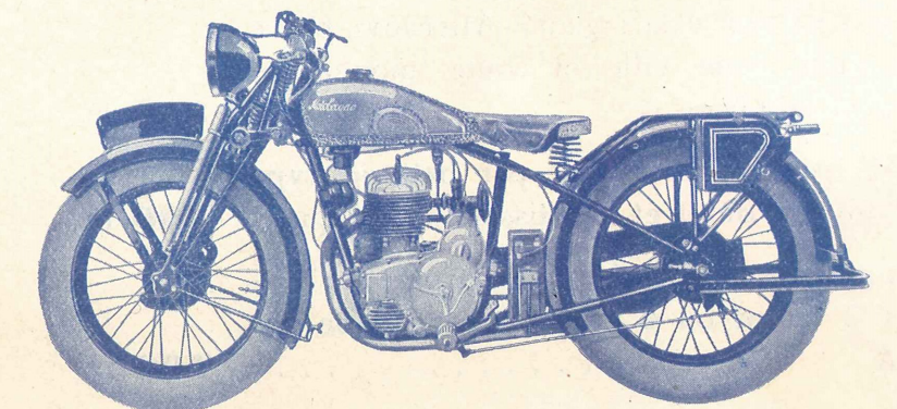
5 CV - 500 cm 3 - Type B 5
