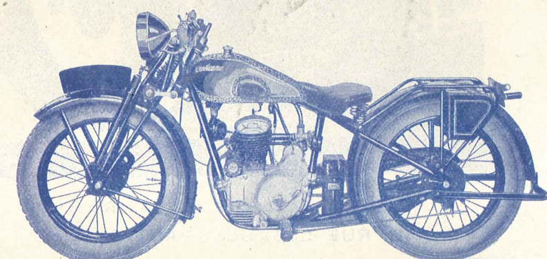
4 CV légère - 350 cm 3 - Type B 44
