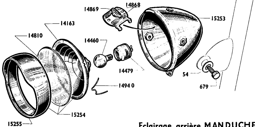
Eclairage arrière MANDUCHER complet 15312
