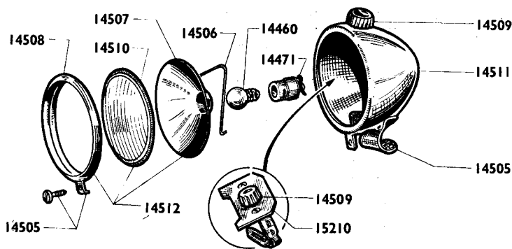
Phare SOUBITEZ 14504
