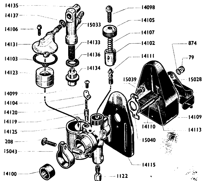
Carburateur complet 15031
