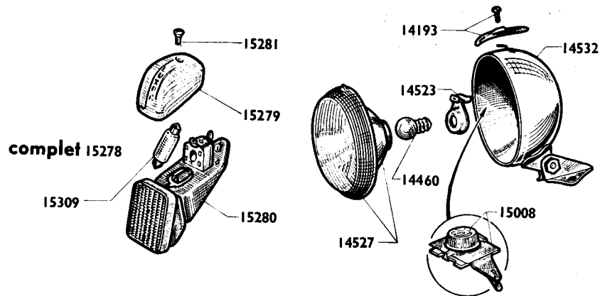
Phare SOUBITEZ 14504
