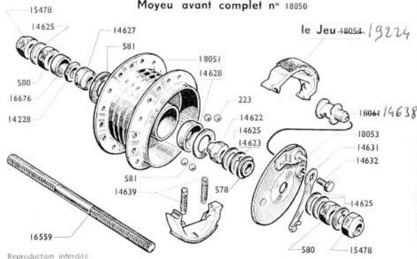
Moyeu avant complet n° 18050
