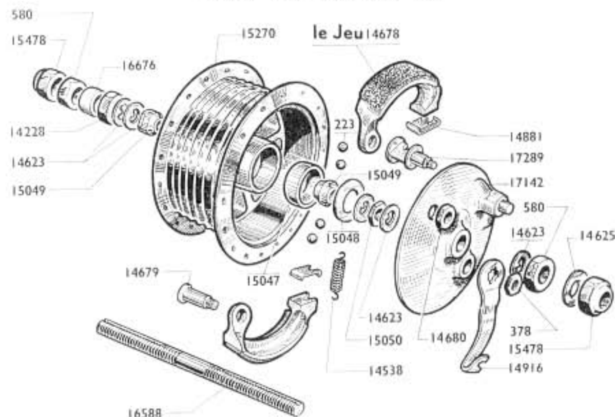
Moyeu avant complet 17140
