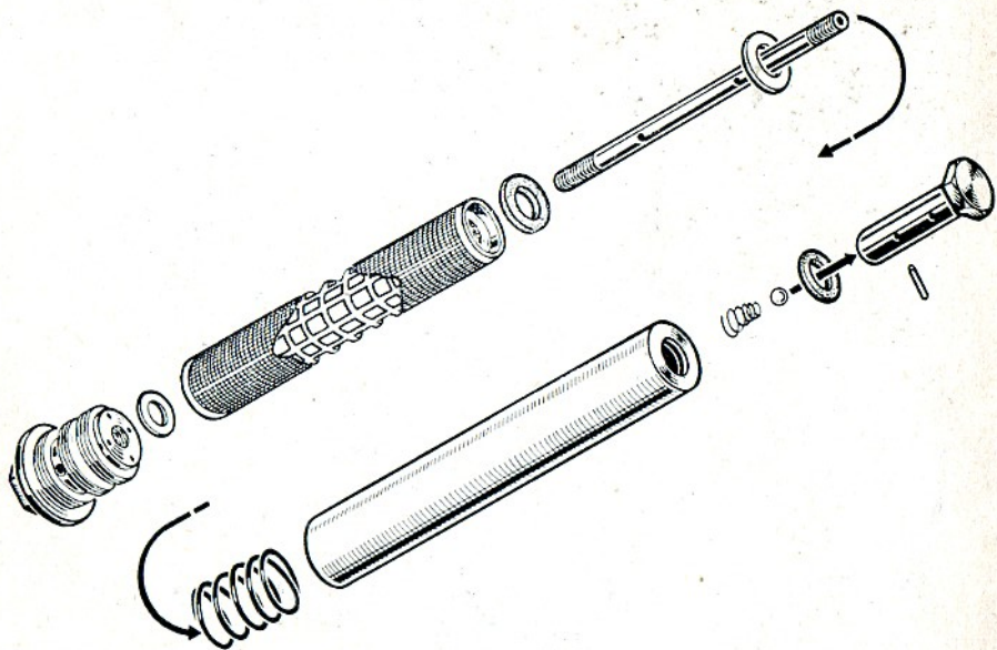
FIGURE N° 6 - Filtre à huile. — Schéma du filtre dans l'ordre de démontage.
