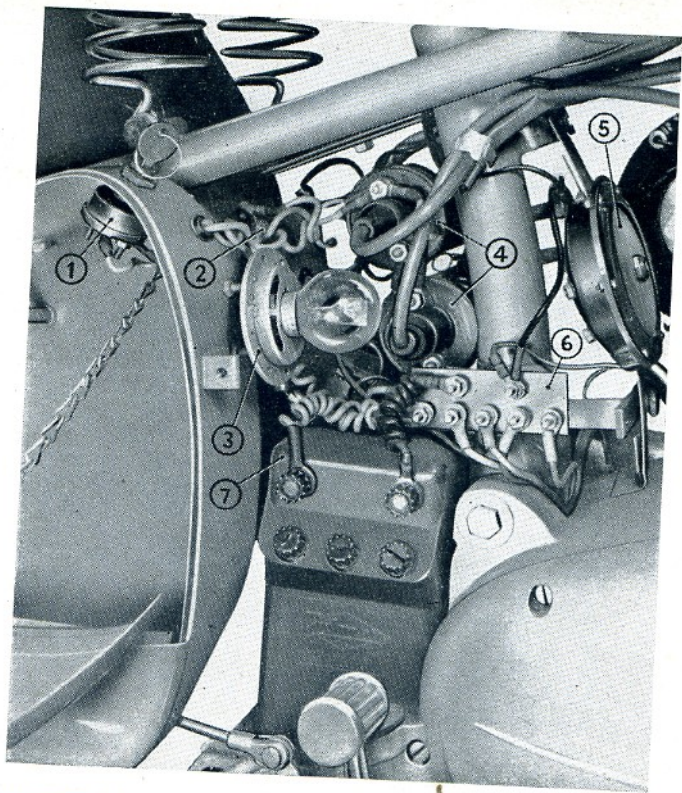
FIGURE N° 4 - Partie du circuit électrique. — 1. Interrupteur de mise en marche. - 2. Cellule redresseuse. - 3. Support et lampe régulatrice. - 4. Bobines d'allumage. - 5. Avertisseur acoustique. - 6. Plaquette relai. - 7. Batterie.
