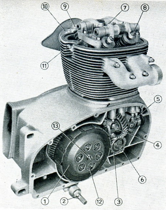
FIGURE N° 3 - BLOC MOTEUR (chapeau de culasse et couvercle embrayage enlevé). — 1. Ensemble embrayage à disques - 2. Arbre de commande du sélecteur. - 3. Pignon de distribution. - 4. Arbre à came. - 5. Poussoir à plateau. - 6. Pignon de commande de pompe à huile. - 7. Culbuterie. - 8. Vis et écrou de réglage des culbuteurs. - 9. Corps du carburateur. - 10. Filtre à air - 11. Bougie. - 12. Écrous de réglage de tension des ressorts de débrayage. - 13. Réglage du débrayage au montage.
